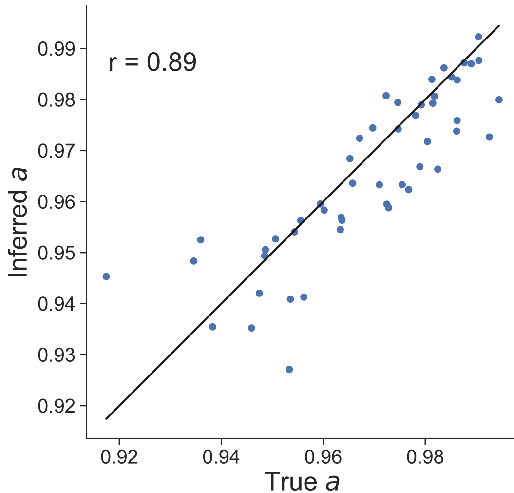
Dataset 12
