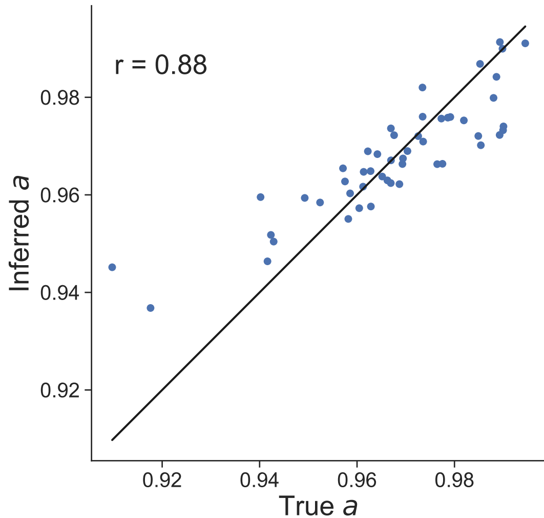
Dataset 13
