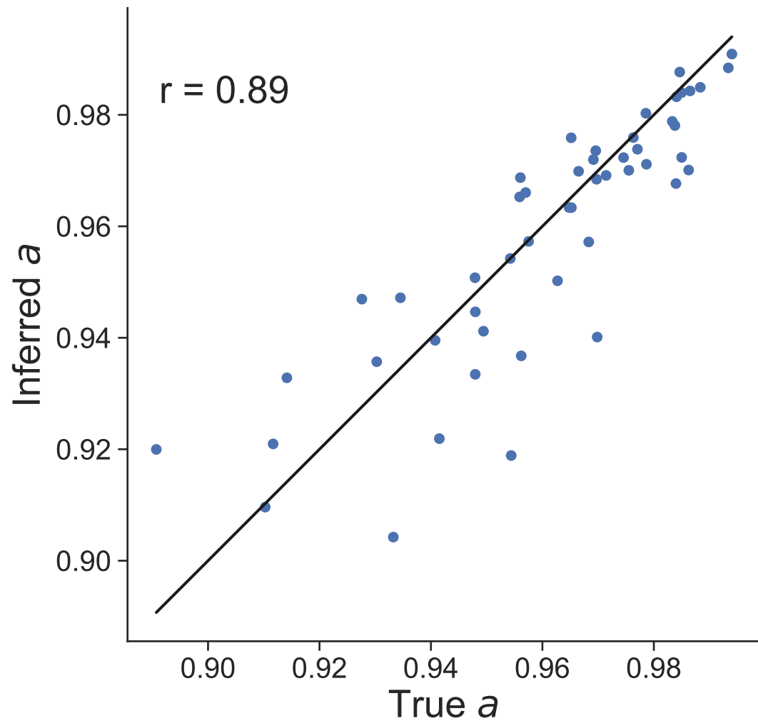
Dataset 32
