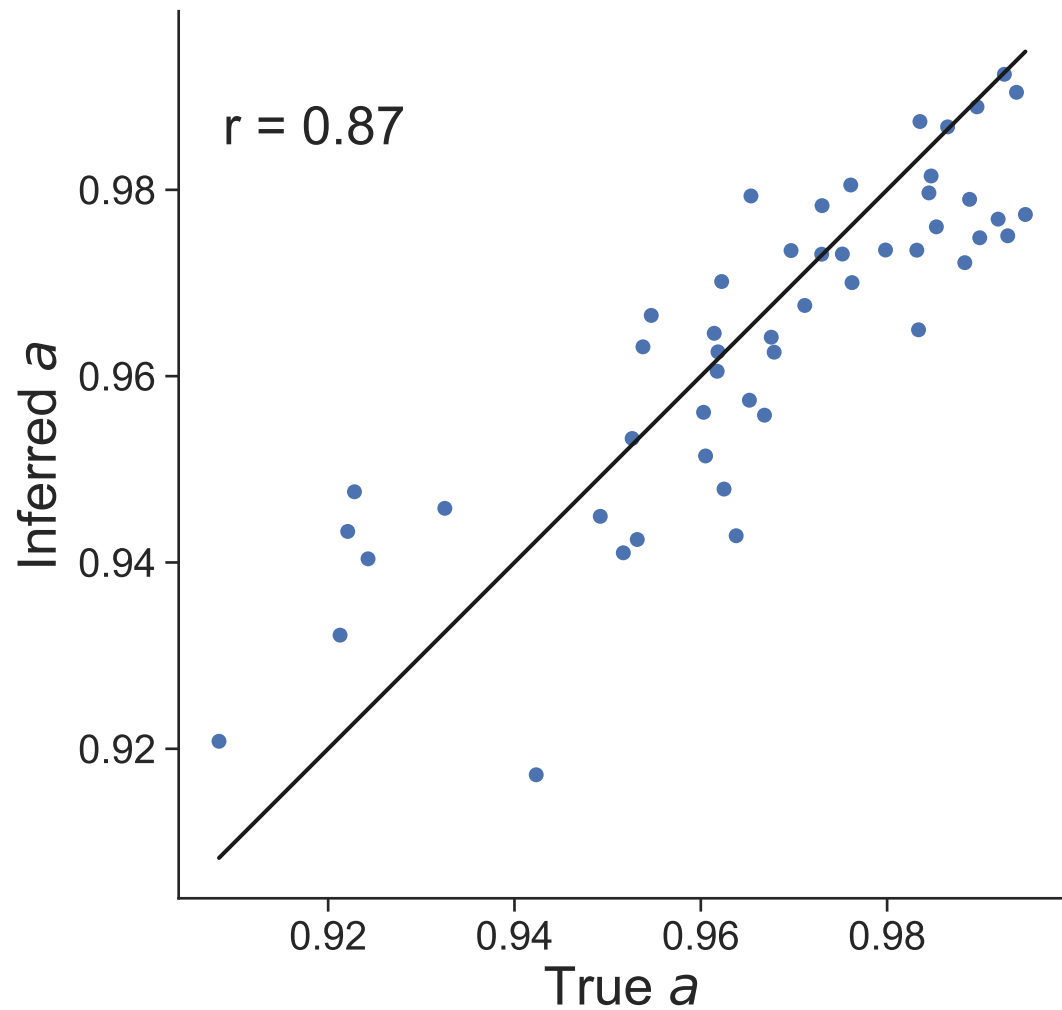
Dataset 1
