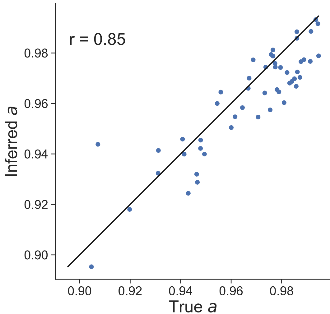
Dataset 42
