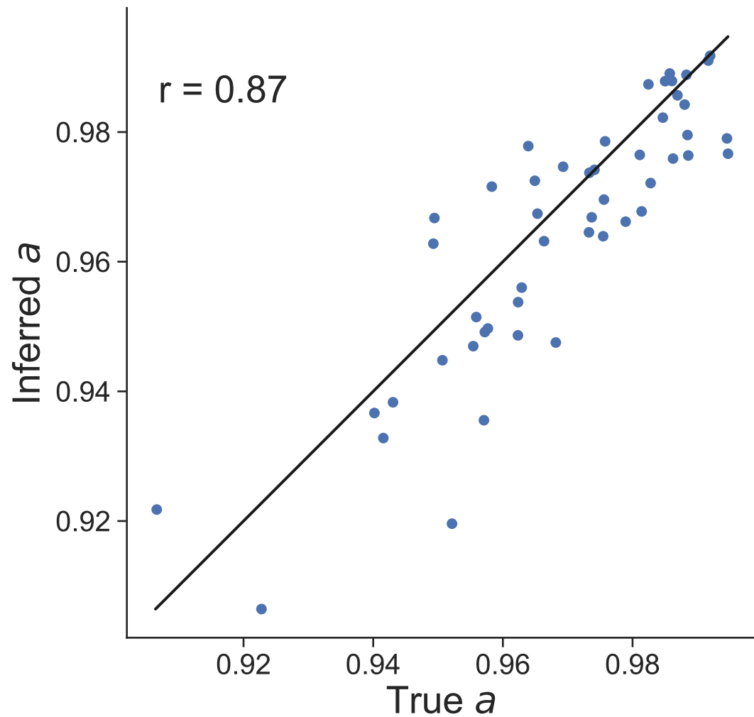
Dataset 29
