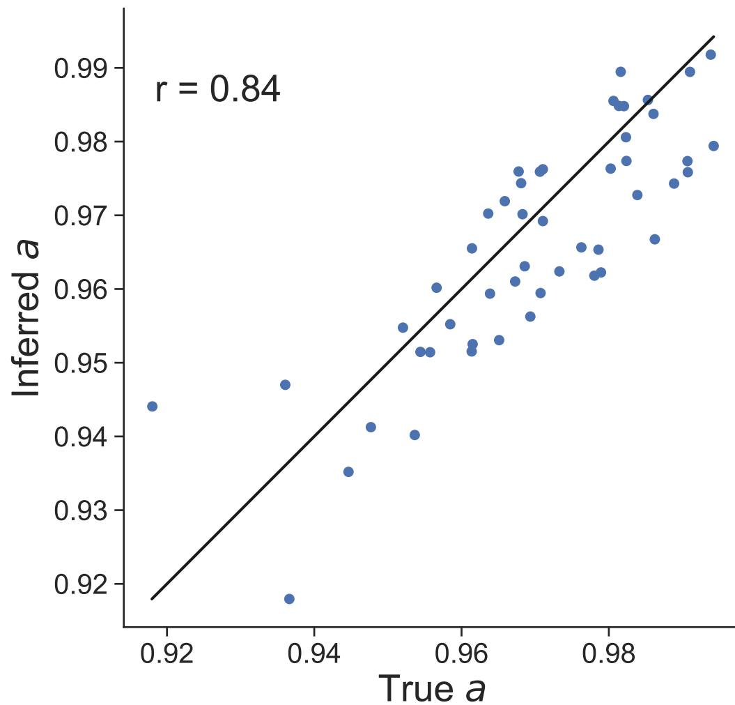
Dataset 4
