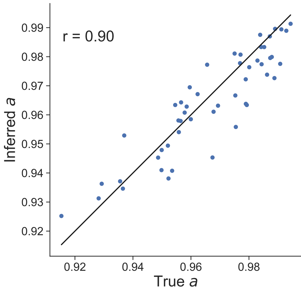
Dataset 45
