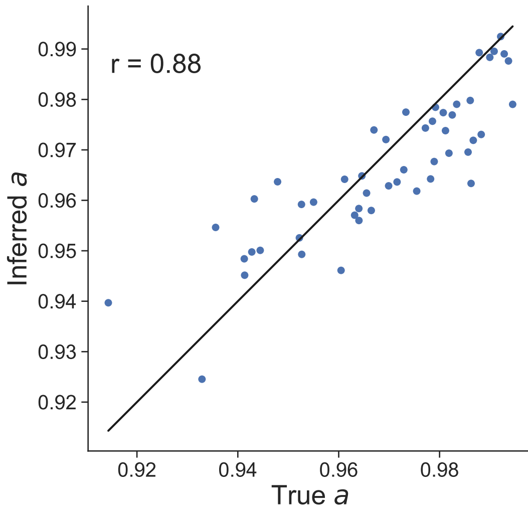
Dataset 21
